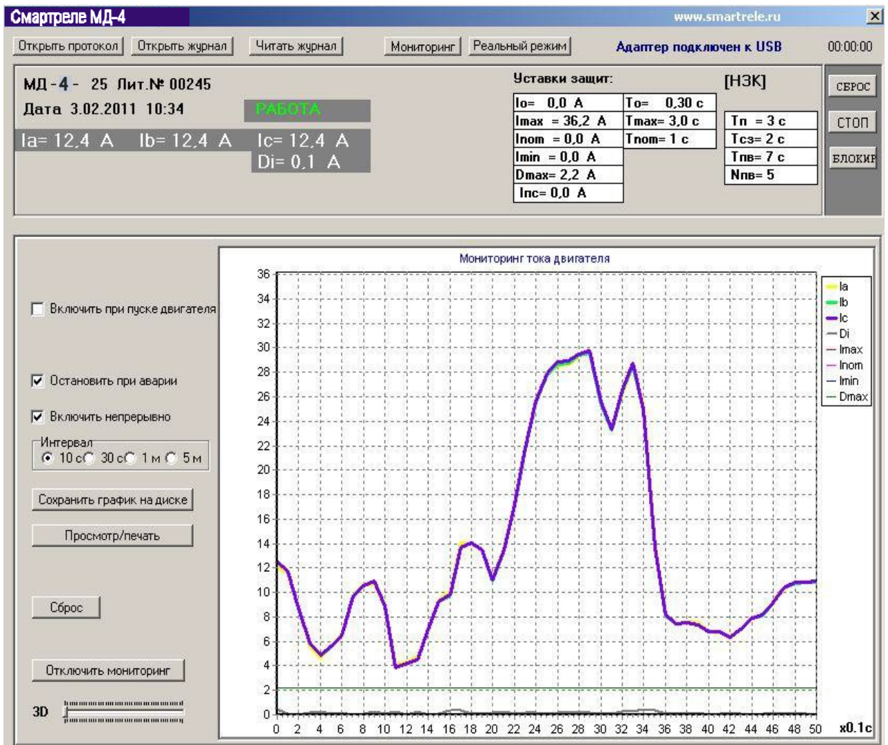
Рисунок 6 – соединение Smartrelе MD-4 с ПК при помощи адаптера USB.
