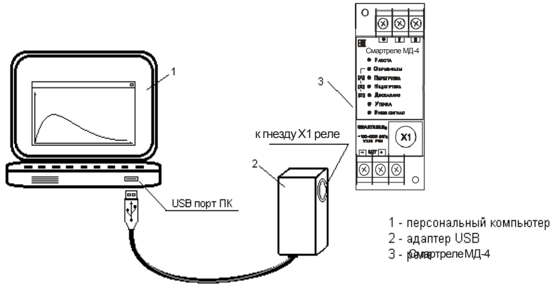
Рисунок 6 – соединение Smartrelе MD-4 с ПК при помощи адаптера USB.
